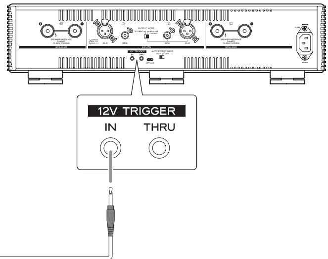
Mono mini-jackplugkabel
